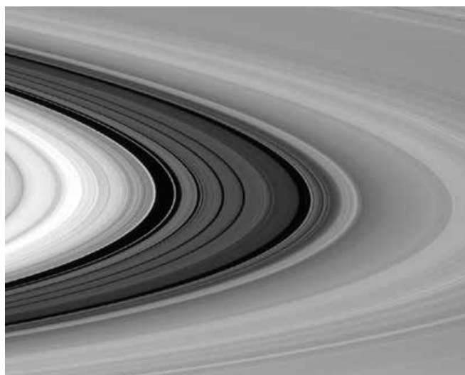
Nærbillede af Cassinis deling, det bredeste af de mørke områder mellem de lyse ringe. Den blev opdaget i 1600-tallet af Giovanni Domenico Cassini, der har givet navn til både delingen og rumsonden, der har taget billedet 28. januar 2017. Foto: NASA/JPL-Caltech/Space Science Institute.
