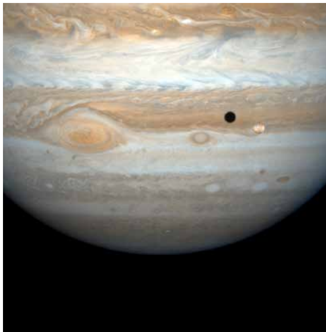
Jupiters måne Io passerer foran planeten og kaster skygge. Billedet er taget fra Cassini rumsonden på vej til Saturn 12. december 2000 fra en afstand på knap 20 millioner km. Foto: NASA/JPL/University of Arizona.
