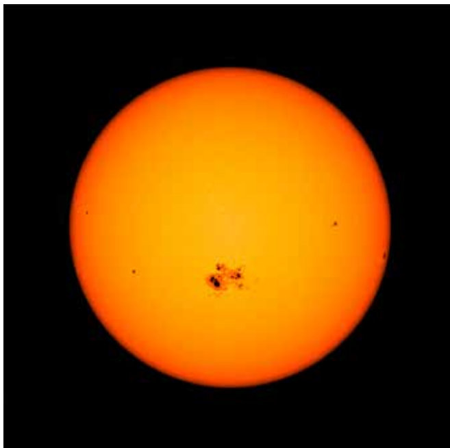
Den største solplet, der er set i en årrække, optaget med NASAs Solar Dynamics Observatory rumsonde 23. oktober 2014. Solpletten fylder næsten 130.000 km, mere end 10 gange Jordens diameter. Den største observerede solplet nogensinde blev set i 1947 og var tre gange så stor. Foto: NASA/SDO.
