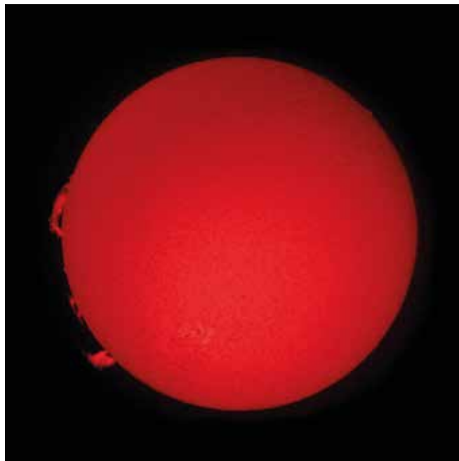
Store protuberanser på Solen optaget gennem Wieth-Knudsen Observatoriets solkikkert i 2015. Foto: Michael Quaade. Billedmanipulation: Rasmus Pape
