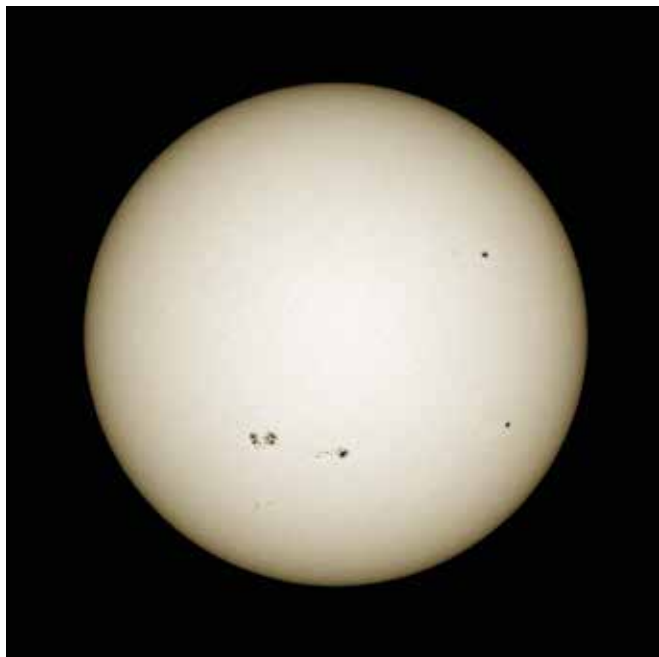
Solpletter optaget 8. september 2021 med Solar Dynamics Observatory satellitten, der har observeret Solen, siden den blev sendt op i 2011. Foto: NASA/SDO and the AIA, EVE, and HMI science teams.
